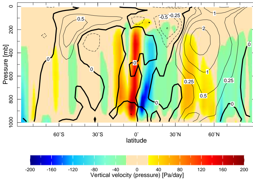
b) omega(colors), u'v'(contours)
